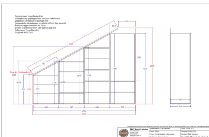
Werktekening met bematingen
